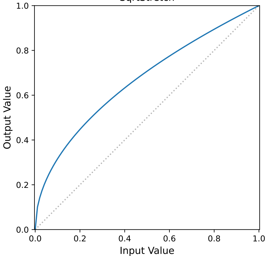
SqrtStretch
